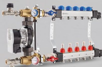
Колектори с дебитомери и функционални вентили и с помпи Wilo Para 25/6 със смесителен елемент - от серия USFP
